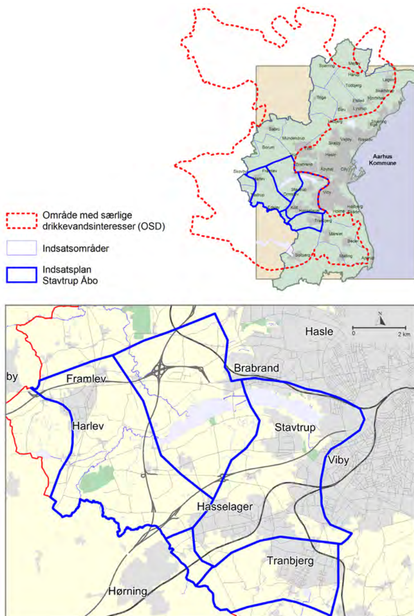
Figur 1. Udstrækningen af OSD, inddelingen i indsatsområder og indsatsområde StautrupÅbo.
