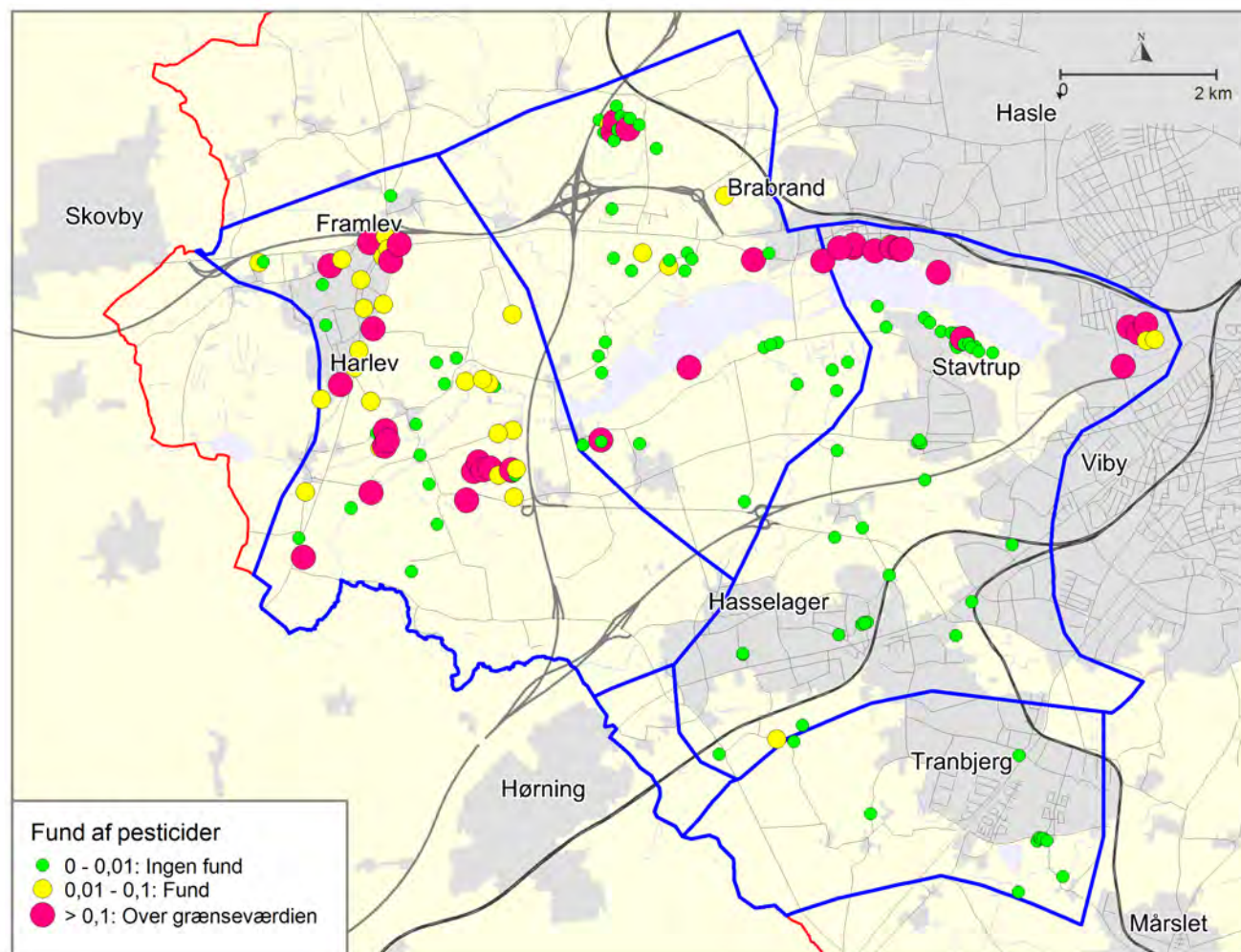
Figur 13. Fund af pesticider i StautrupÅbo indsatsområde. Koncentrationer er angivet i µg/l.
