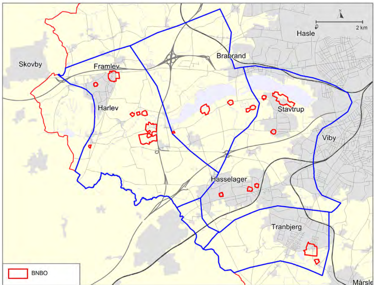
På figur 9 vises BNBO omkring indvindingsboringer til almene vandværker i indsatsområdet.
