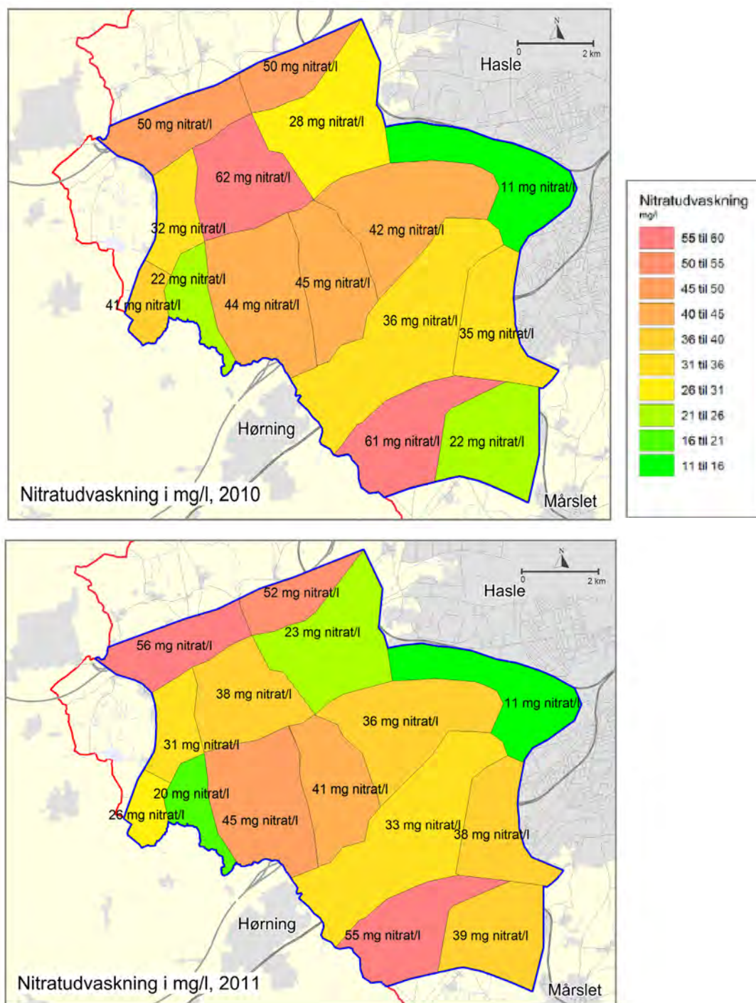
Figur 4. Udvasningen af nitrat i gennemsnit for hvert delopland beregnet på baggrund af indberettede dyrkningsoplysninger for 2010 og 2011.
