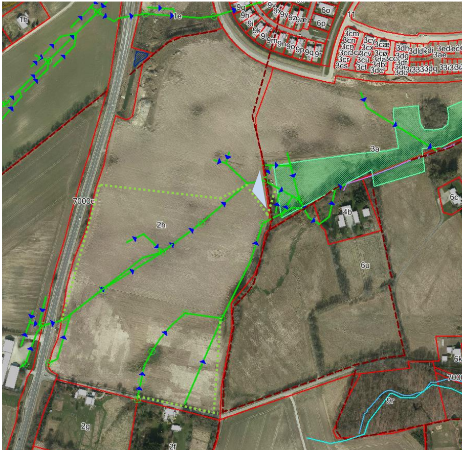
Figur 2: Projektforslag: Omlagte dræn: ..... / Bassin: ▲
