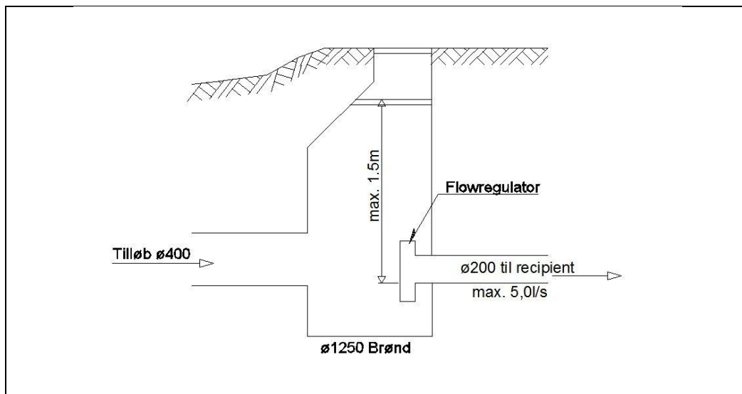
Figur 4.1 Brønd med regulator (se eksempel 3).
