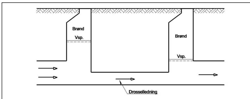
Figur 2.4 Drosselledning.
