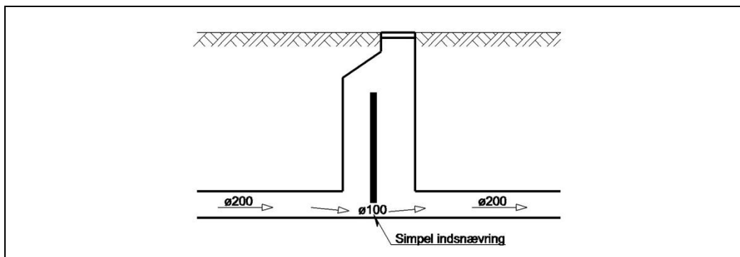
Figur 2.3 Simpel punktindsnævring.
