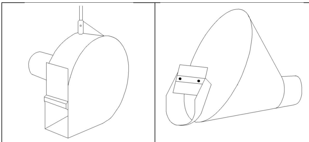
Figur 2.5 Centrifugalbremse til venstre og cyklonbremse til højre.
