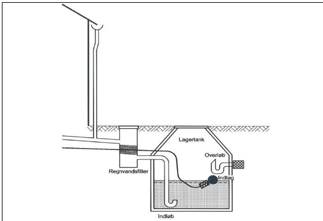
Figur 3.3 Skitse af lagertankens indvendige udformning.
