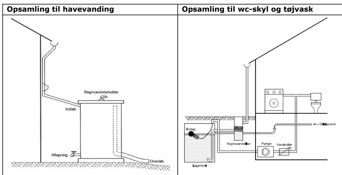
Figur 1.1 Eksempel på opsamling af regnvand.
